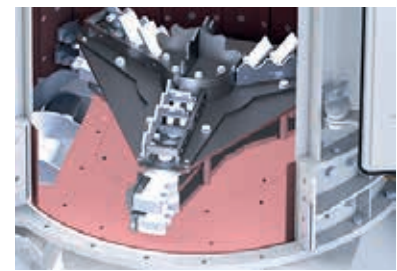
C Einfach zu wechselnde Schläger und Prallteile
