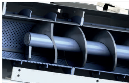
A Vis tournant dans un cylindre perforé comprimant les inertes
