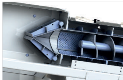
B Obturateur réglable sous la pression des inertes en sortie de vis
